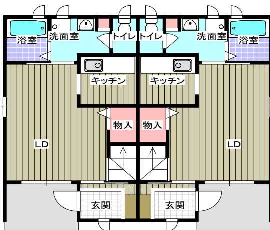
101 ▼1階 102
